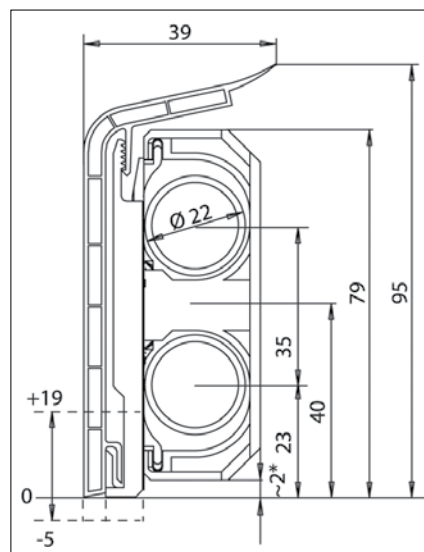
Przekrój montażu listwy SLF
