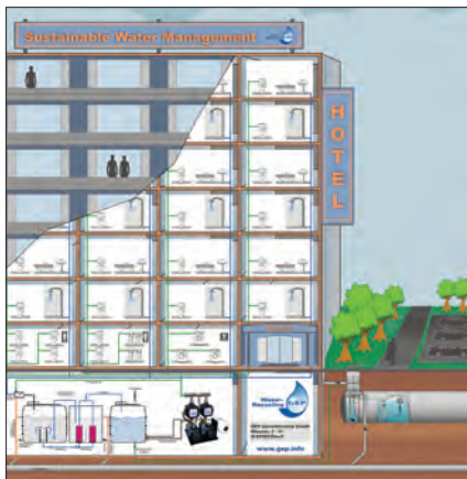
System przetwarzania i wykorzystania wody szarej
